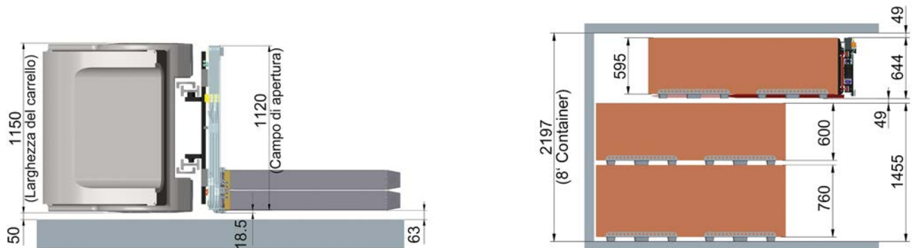
Vista dall'alto 2T163S/ST
